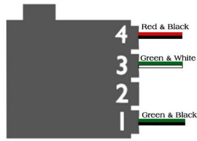
UD6089 (4 Pin)
