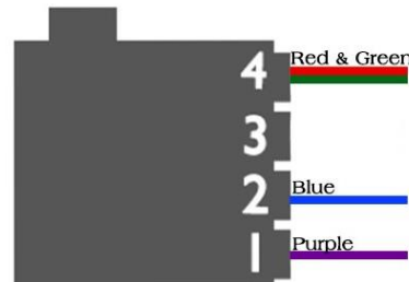
UD6089 (4 Pin)
