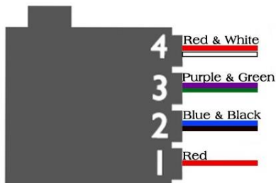
UD6089 (4 Pin)
