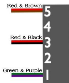
RH13253 (5 Pin)
